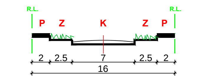
PRESJEK B1-B1
