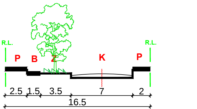
PRESJEK D-D
