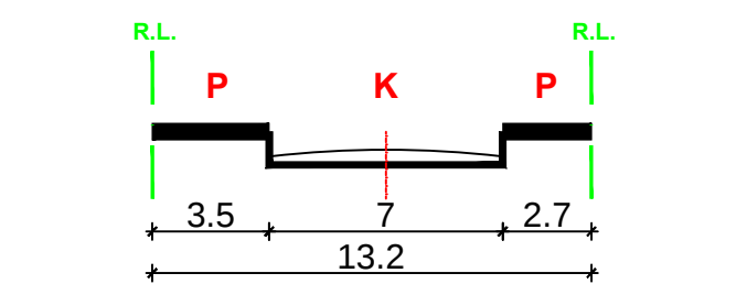
PRESJEK B-B
