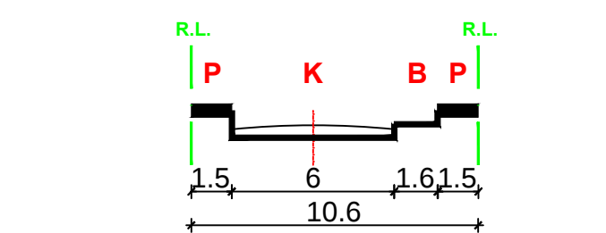
PRESJEK E1-E1
