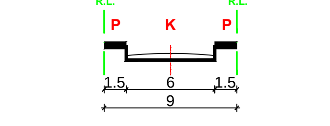
PRESJEK E-E
